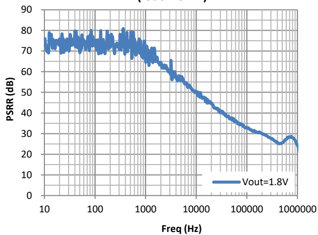
PSRR (Iout=10mA)
