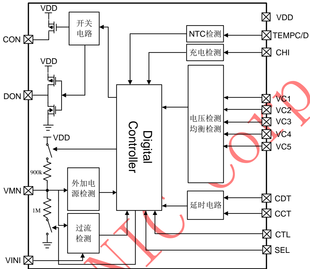
图 2 IP3259 功能框图
